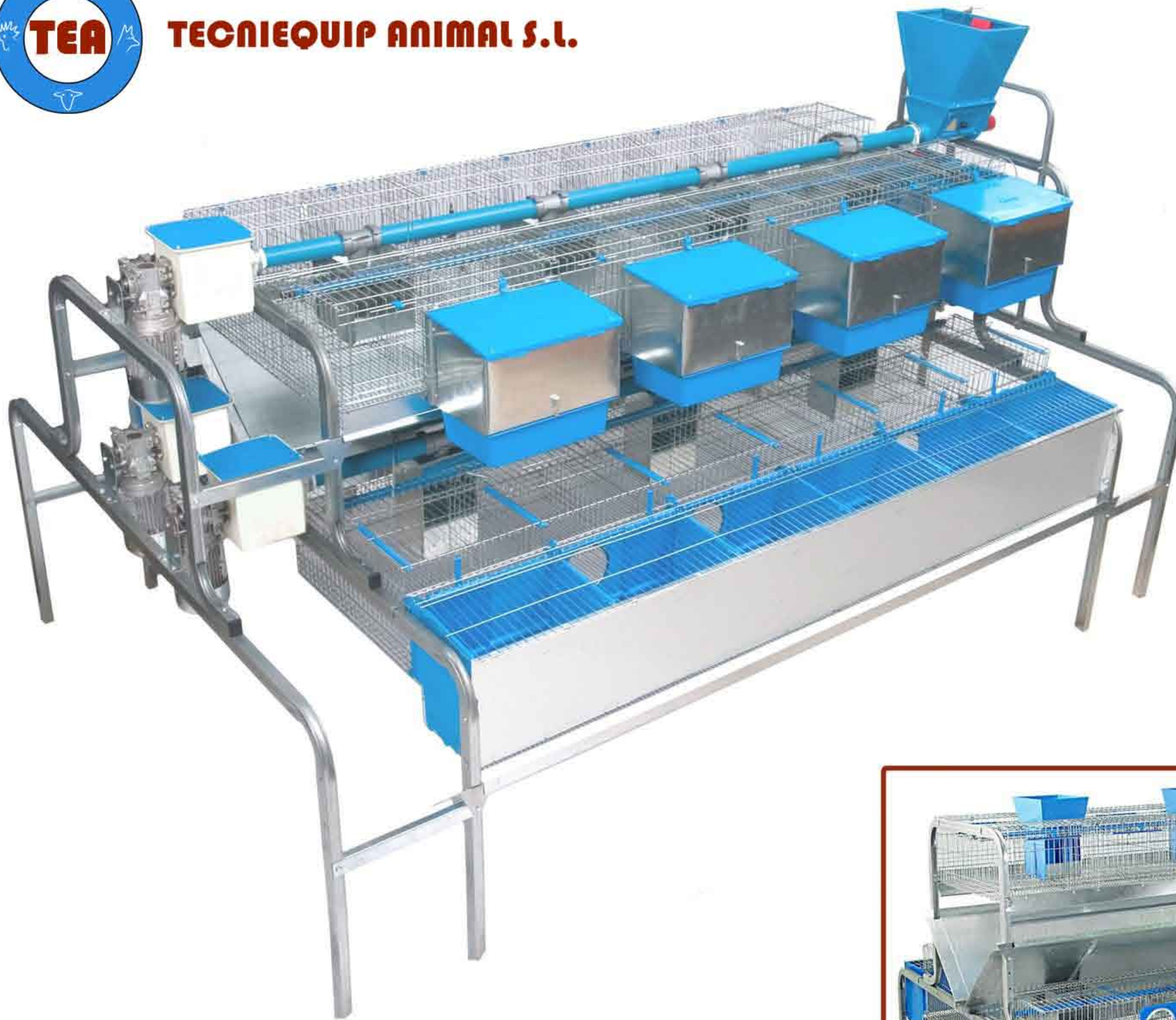
E.3 MODULO MEGA BABY 12/16 6/4-T F2000 CON ALIMENTACION AUTOMATICA
