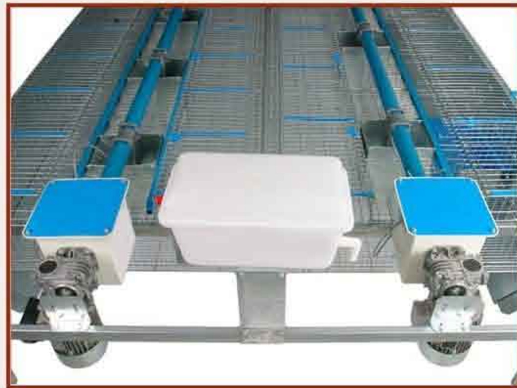
INICIO ALIMENTACION DOBLE CENTRAL E.3 2400 Ref.40.12003
